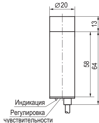
Габаритный чертёж
