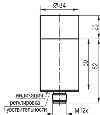
Габаритный чертеж
