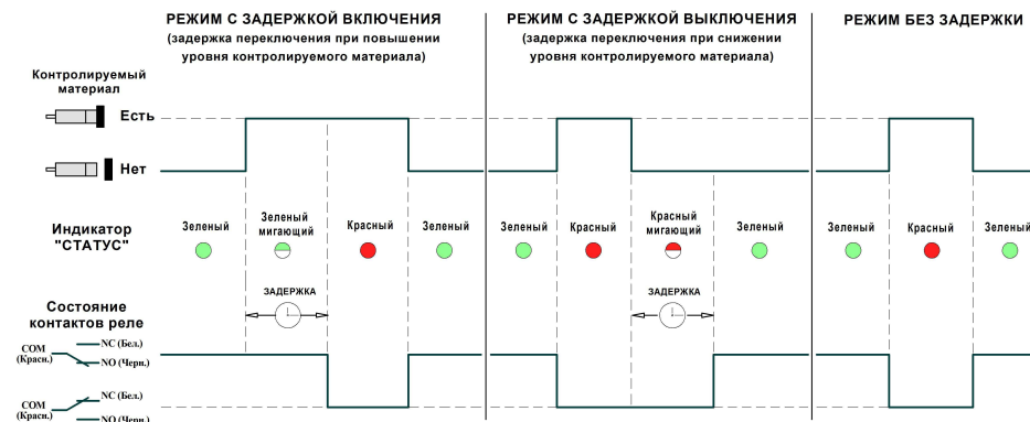
Рис.2 - Диаграммы работы датчика
