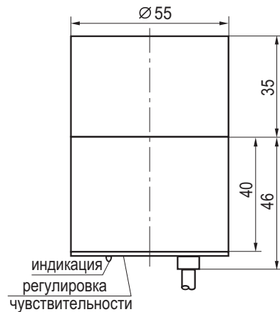
Габаритный чертёж
