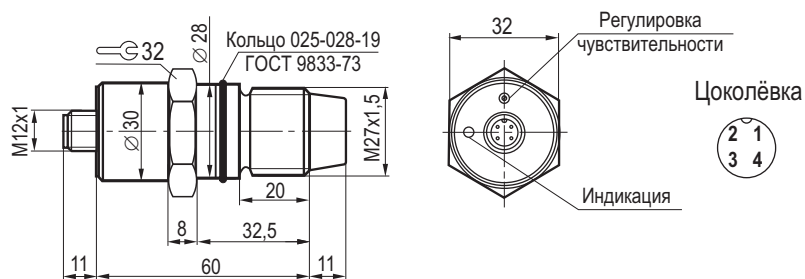
Габаритный чертёж
