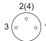
Цоколевка соединителя CP S401 (вид со стороны монтажа)
