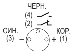
Цоколевка соединителя CS S15-1-2
