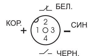
Цоколевка соединителя CS S19-3-
