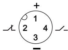
Цоколевка соединителя CS S25-3 (вид со стороны монтажа)
