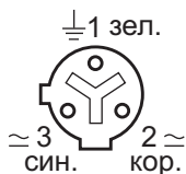
Цоколевка соединителя CS S27-
