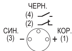
Цоколевка соединителя CS S48-1-
