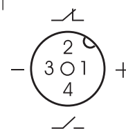
Цоколевка соединителя CS SF254-3 (вид со стороны монтажа)
