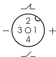
Цоколевка соединителя CS SF254-3 (вид со стороны монтажа)
