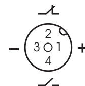
Цоколевка соединителя CS SF255-3 (вид со стороны монтажа)
