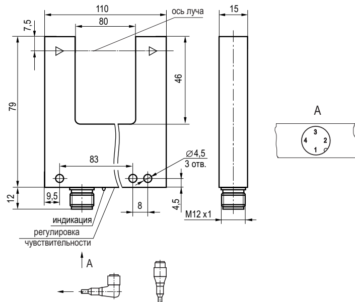
Габаритный чертёж
