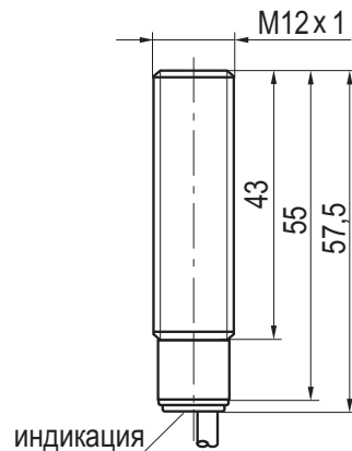
Габаритный чертёж
