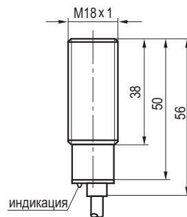
Габаритный чертеж
