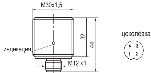
Габаритный чертеж
