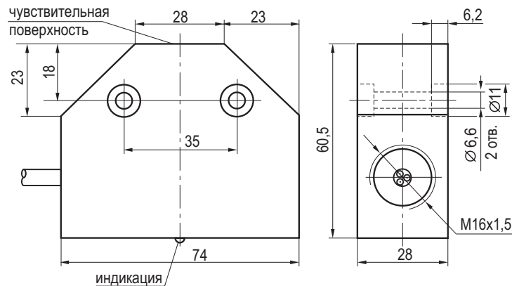
Габаритный чертёж
