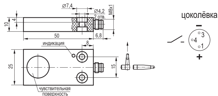
Габаритный чертёж
