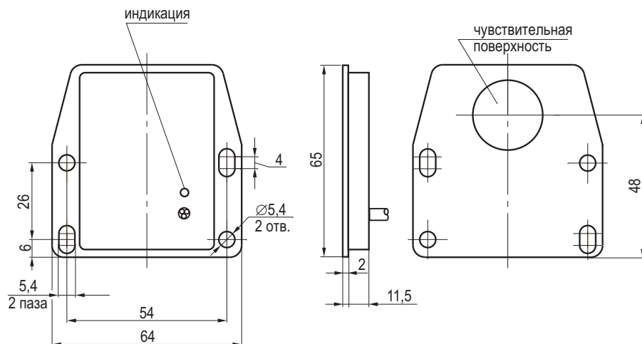
Габаритный чертёж
