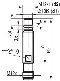
Габаритный чертеж
