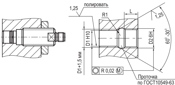
Схема монтажа
