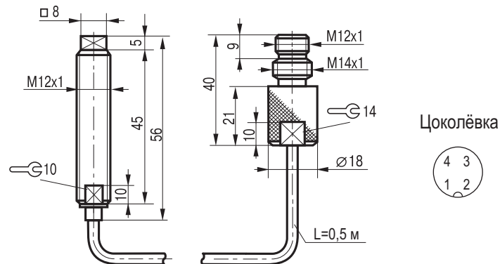
Габаритный чертёж
