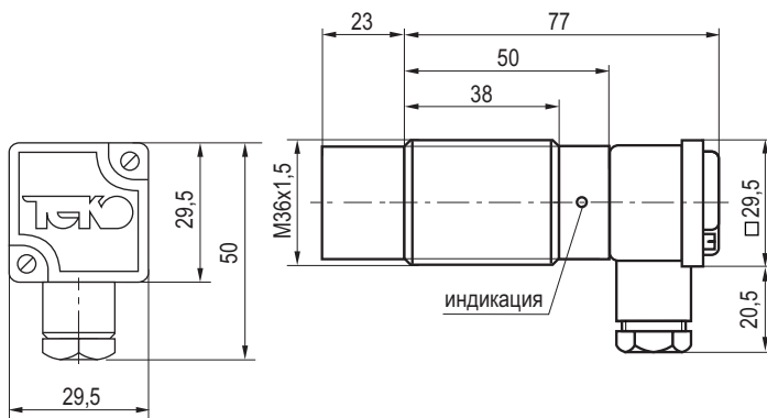
Габаритный чертёж
