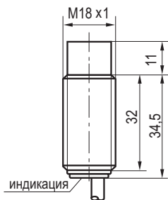
Габаритный чертеж
