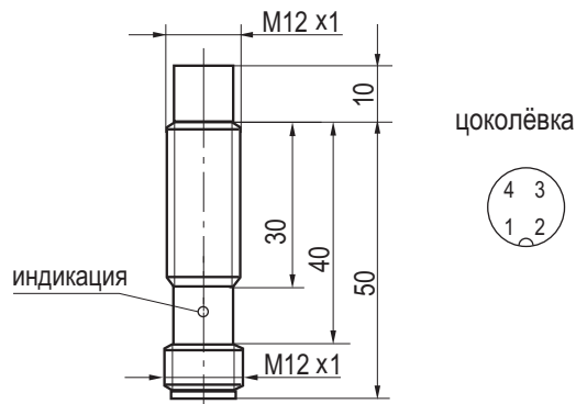
Габаритный чертёж
