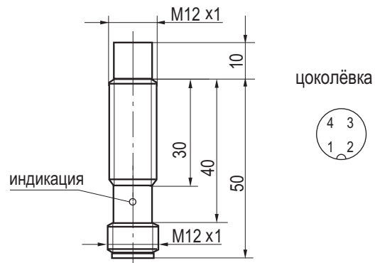
Габаритный чертёж
