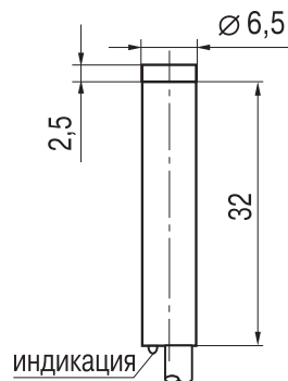
Габаритный чертёж
