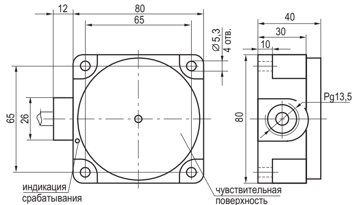
Габаритный чертеж
