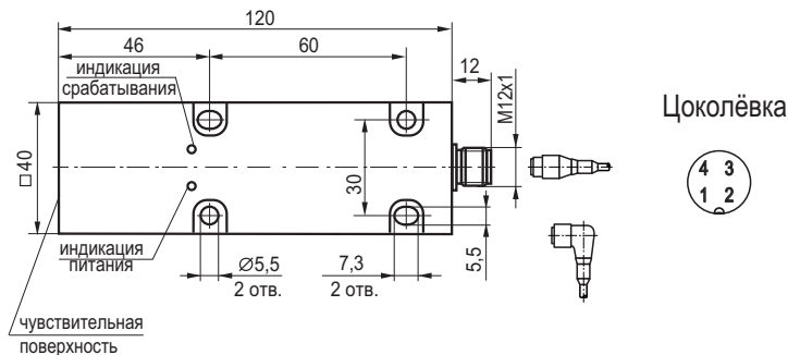
Габаритный чертёж
