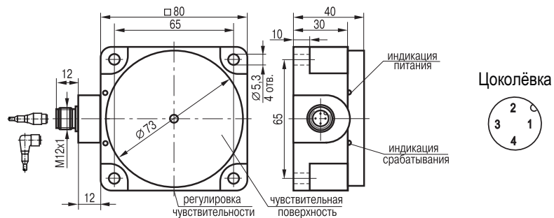
Габаритный чертёж
