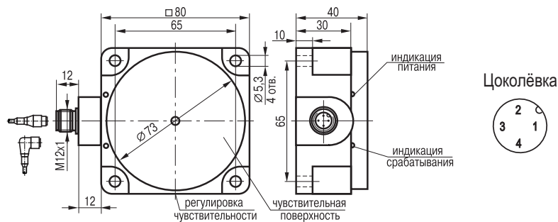
Габаритный чертеж
