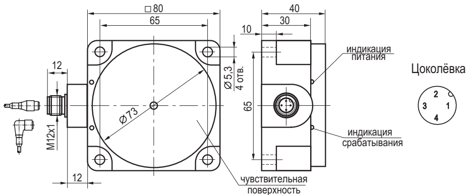
Габаритный чертёж
