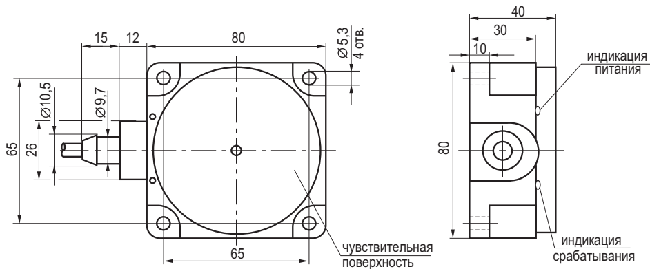
Габаритный чертёж
