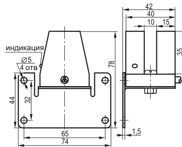
Габаритный чертёж
