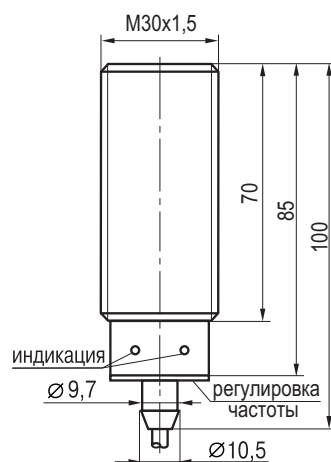
Габаритный чертёж
