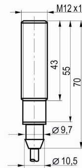
Габаритный чертеж
