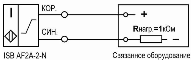
Схема подключения к оборудованию
