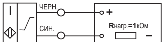
Схема подключения к оборудованию
