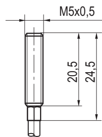
Габаритный чертеж
