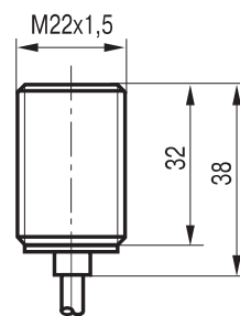
Габаритный чертеж
