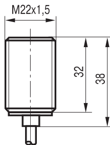
Габаритный чертеж
