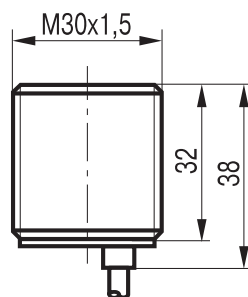
Габаритный чертеж
