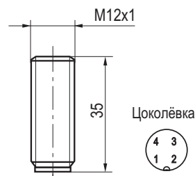
Габаритный чертеж
