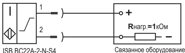
Схема подключения к оборудованию
