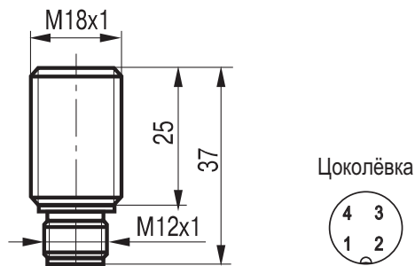
Габаритный чертеж
