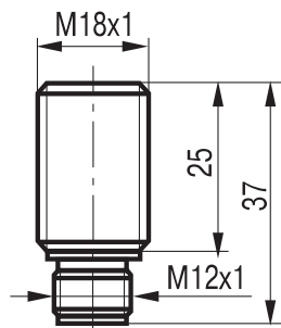
Габаритный чертеж
