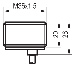
Габаритный чертеж
