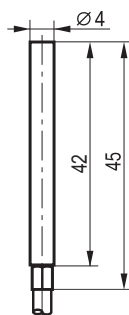
Габаритный чертеж
