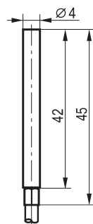
Габаритный чертеж
