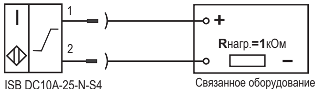
Схема подключения к оборудованию
