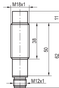
Габаритный чертеж
