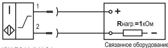
Схема подключения к оборудованию
